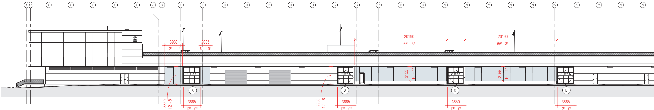
ÉLÉVATION SUD - PARTIE 1 / ELEVATION SOUTH - PART 1
