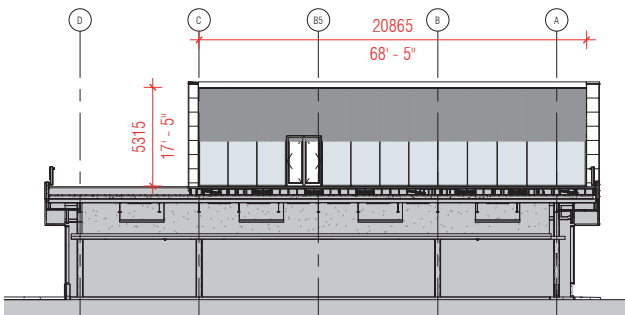
ÉLÉVATION OUEST - PAVILLON / ELEVATION WEST - PAVILLON
