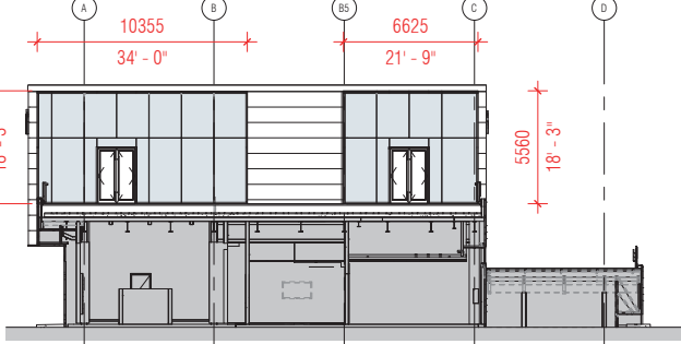
ÉLÉVATION EST - PORT CENTRE / ELEVATION EAST - PORT CENTRE
