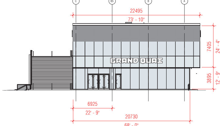
ÉLÉVATION OUEST - CÔTÉ PROMENADE DU VIEUX PORT / ELEVATION WEST - PROMENADE DU VIEUX PORT SIDE
