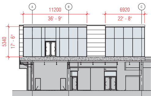
ÉLÉVATION EST - PAVILLON / ELEVATION EAST - PAVILLON
